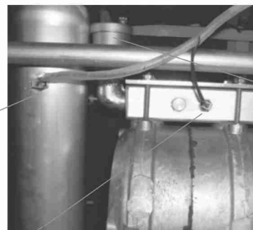
Автоматический воздухоотводчик
